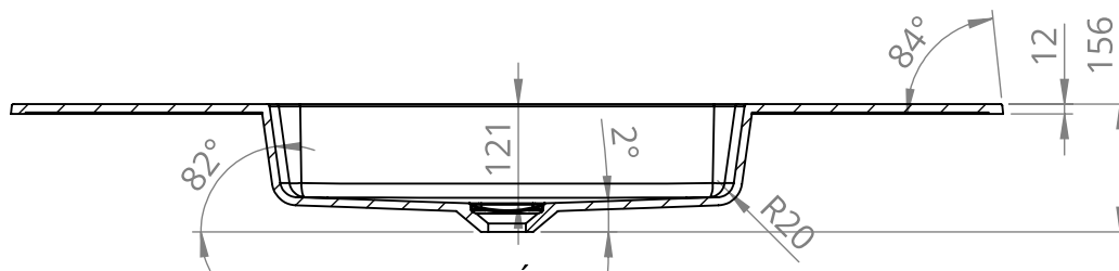
PRZEKRÓJ G-G SKALA 1 : 10
